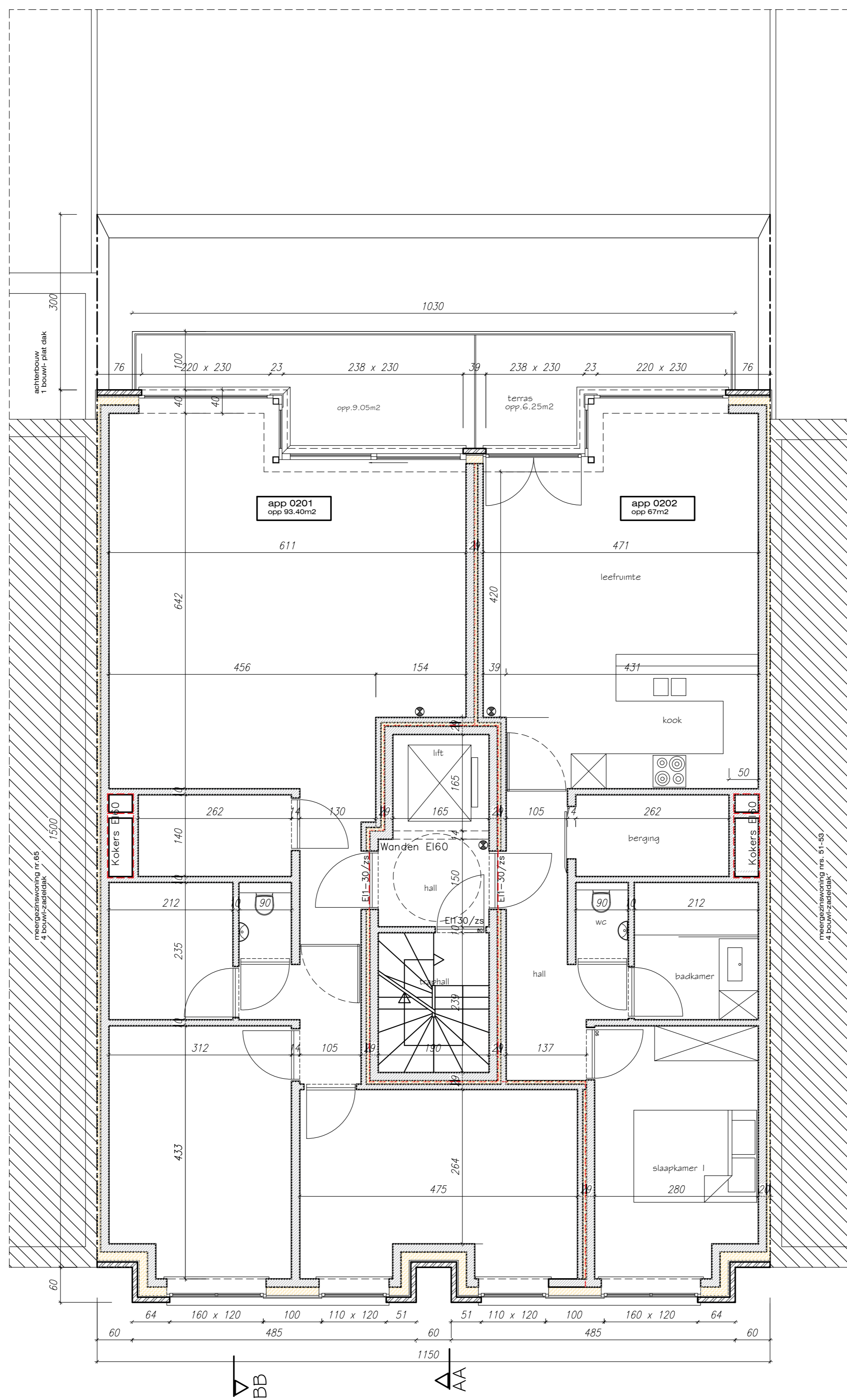
RESIDENTIE IGUAZU VERDIEPING 2 APP. 0201 APP. 0202
