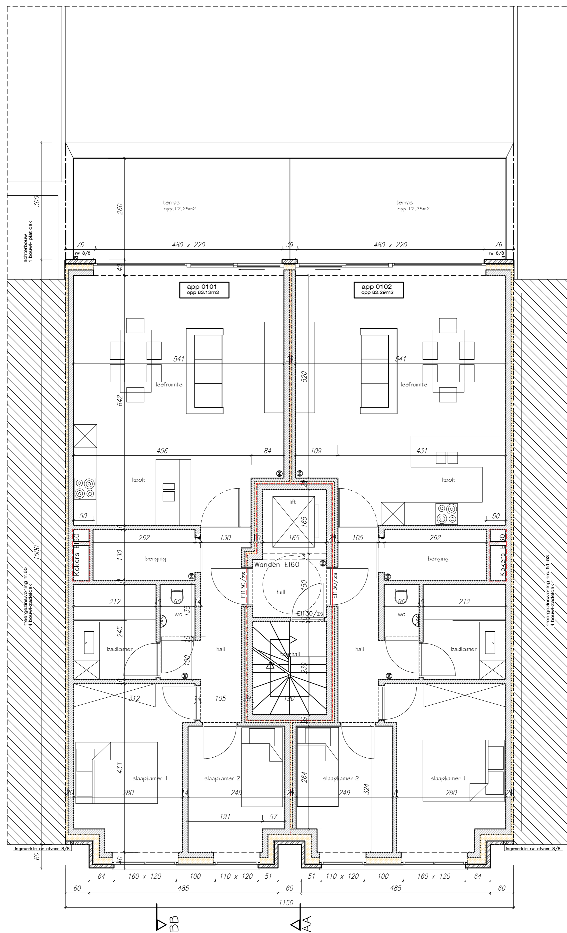
RESIDENTIE IGUAZU VERDIEPING 1 APP. 0101 APP. 0102
